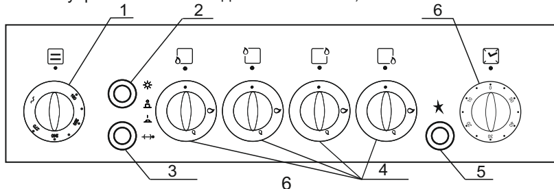
Панель управления плит моделей 506040.01г, 506040.11г
