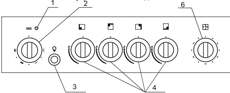
Панель управления плит модели 5040.41гэ
